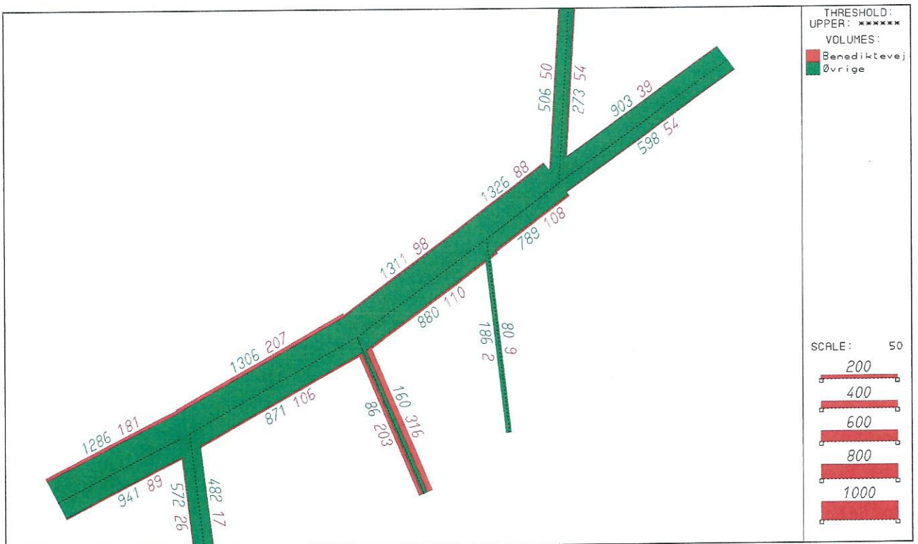
Figur 6 Gennemkørende trafik til/fra Benediktevej vist med rødt og øvrig trafik på vejene vist med grønt
