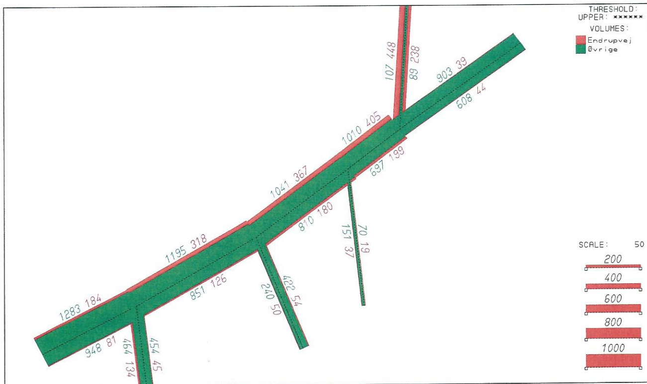
Figur 3 Gennemkørende trafik til/fra Endrupvej vist med rødt og øvrig trafik på vejene vist med grønt
