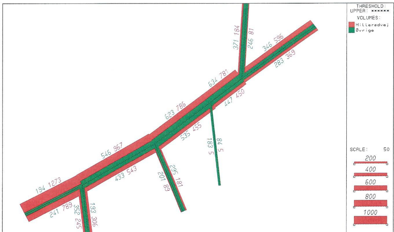
Figur 8 Gennemkørende trafik til/fra Hillerødvej vist med rødt og øvrig trafik på vejene vist med grønt
