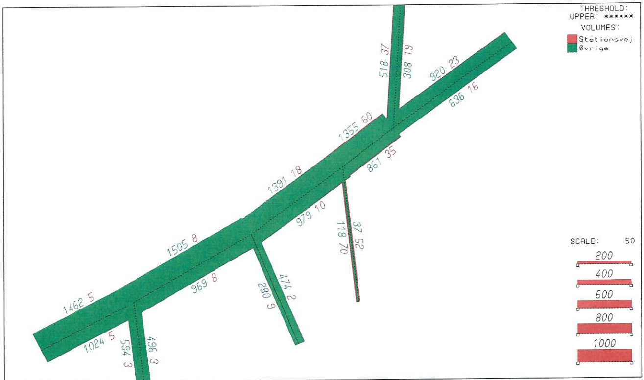
Figur 5 Gennemkørende trafik til/fra Stationsvej vist med rødt og øvrig trafik på vejene vist med grønt
